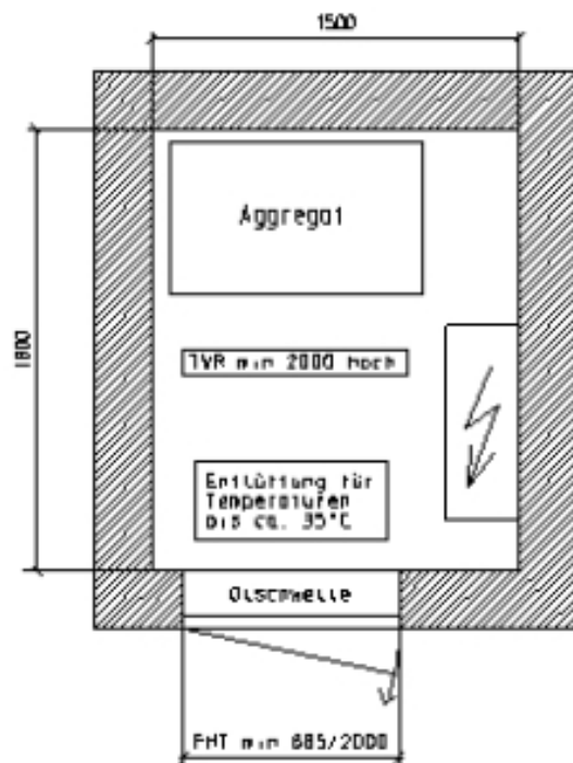
Triebwerksraumgrundriß
