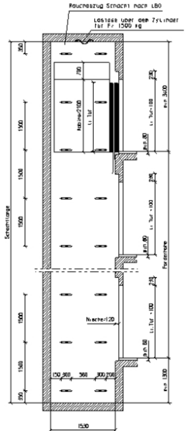
Schnitt A-A
