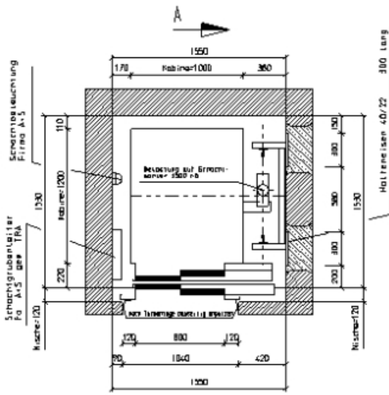
Schachtgrundriß
